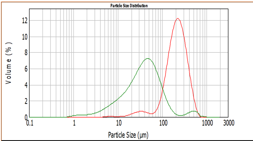
Raspodela veličina čvrstih čestica u ekstraktima (— ekstrakt Cognivia™, — ekstrakt acerole)
